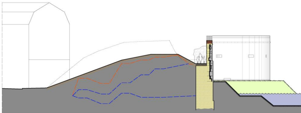
Doorsnede vergunningaanvraag. De fijne, zwarte stippellijn toont de huidige doorsnede van de wal; de gekleurde stippellijnen daaronder laten de diverse archeologische lagen van de aarden wal zien. Bron: HVN architecten
